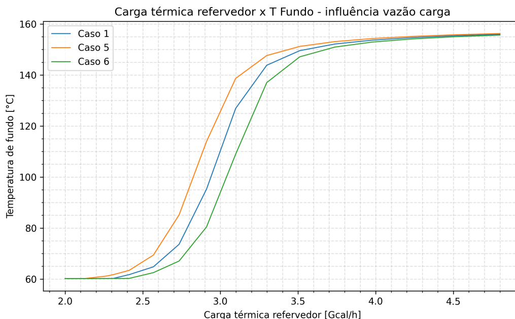
Figura 6: Carga térmica x temperatura do fundo - Influência Vazão da Carga
